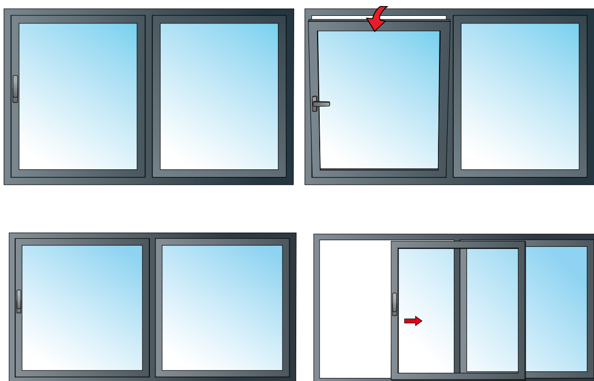
g) okno uchylno-przesuwne
